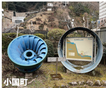
小国町の杖立温泉に立ち寄った時、旧杖立発電所(水力発電)で使用されていた水車と水圧鉄管の展示を見ました。両方とも精密に作られた迫りがありました。杖立温泉には水力と温泉熱発電所があり、約1800年の歴史ある温泉地は、今日も癒しとエネルギーを生み出しています。K/S
